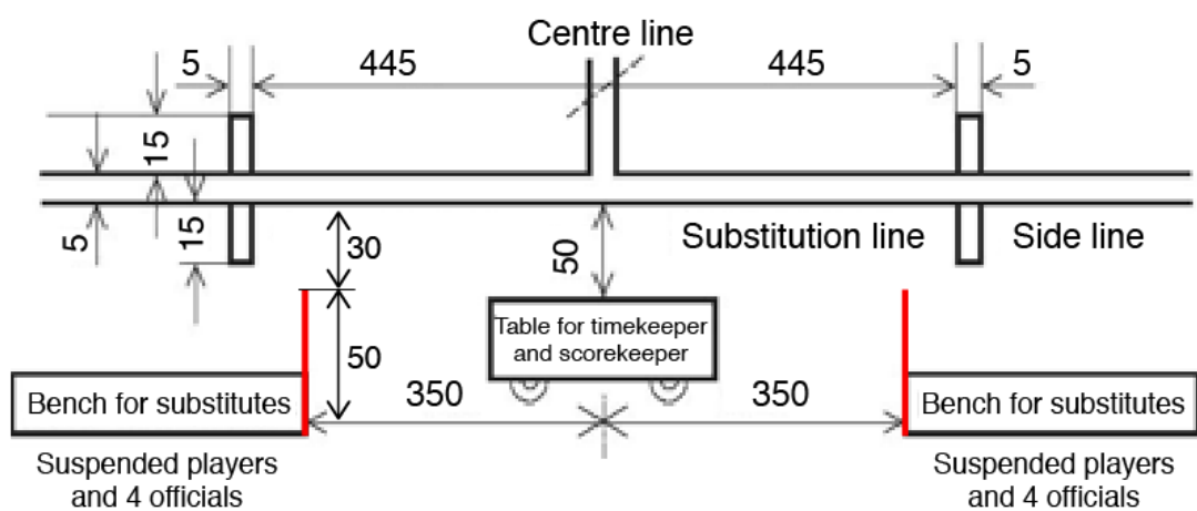
Figuur 3: Wisselijnen en wisselzones
